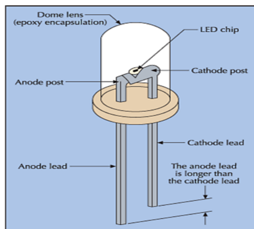
شکل ۱: ساختار یک LED
